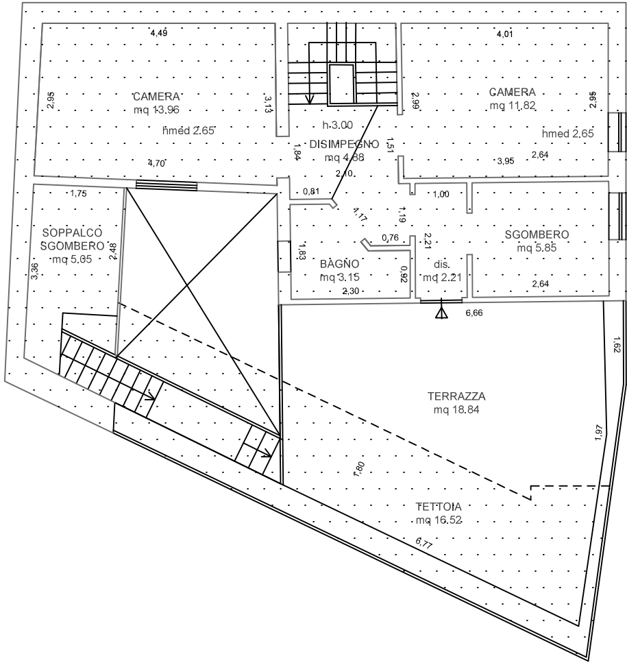
PIANO PRIMO
